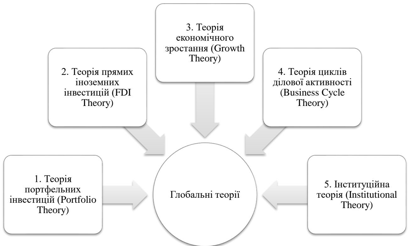
Рис. 1.1 Глобальні теорії
