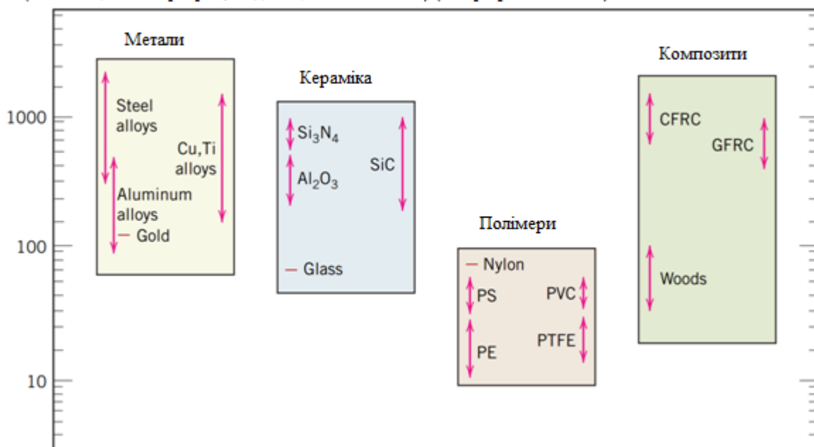
Рис. 1.5. Гістограма значень міцності, при кімнатній температурі (тобто міцності на розрив), для різних металів, кераміки, полімерів і композитних матеріалів.
