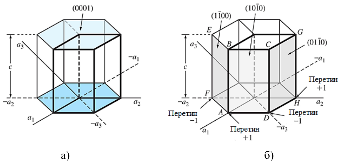
Рис. 3.16. Індеси Міллера-Браве гексагональних кристалічних площин: а) – базисних площин; б) – площин призм.
