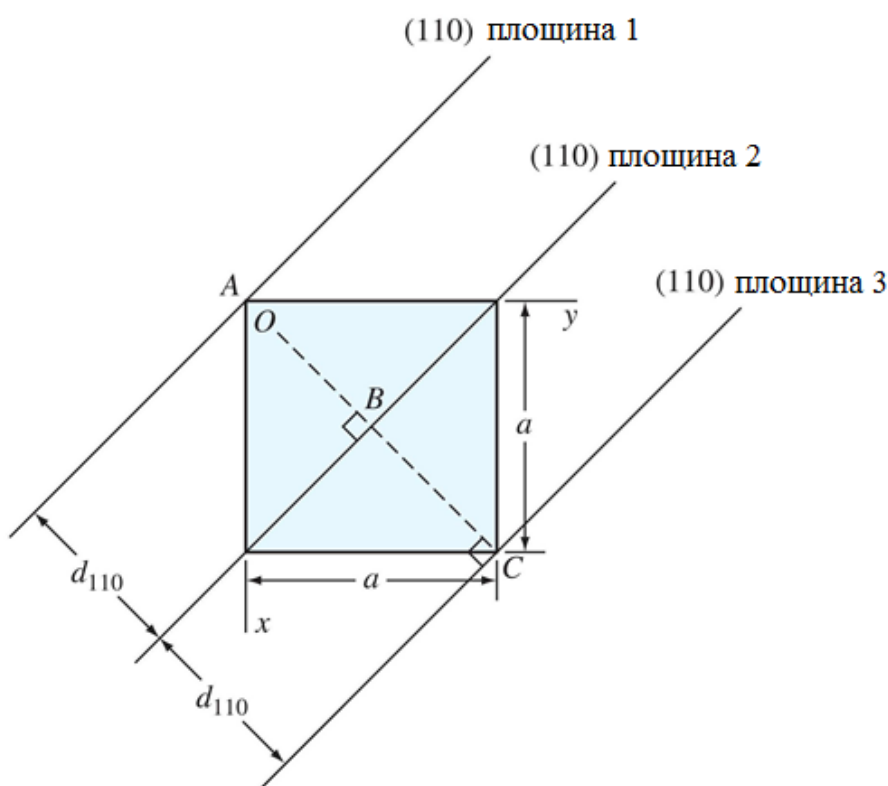
Рис. 3.14. Вид зверху кубічної елементарної комірки, що показує відстань між (110) кристалічними площинами, d_{110} .
