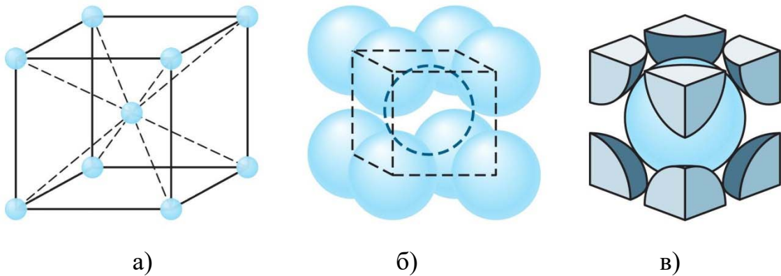
Рис. 3.5. Елементарні комірки ОЦК ґратки: а) – елементарна комірка з атомними вузлами; б) – елементарна комірка з твердою сферою; в) – ізольована елементарна комірка.
