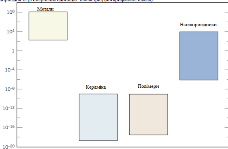
Електропровідність (в обернених одиницях ом-метрів) (логарифмічна шкала)
