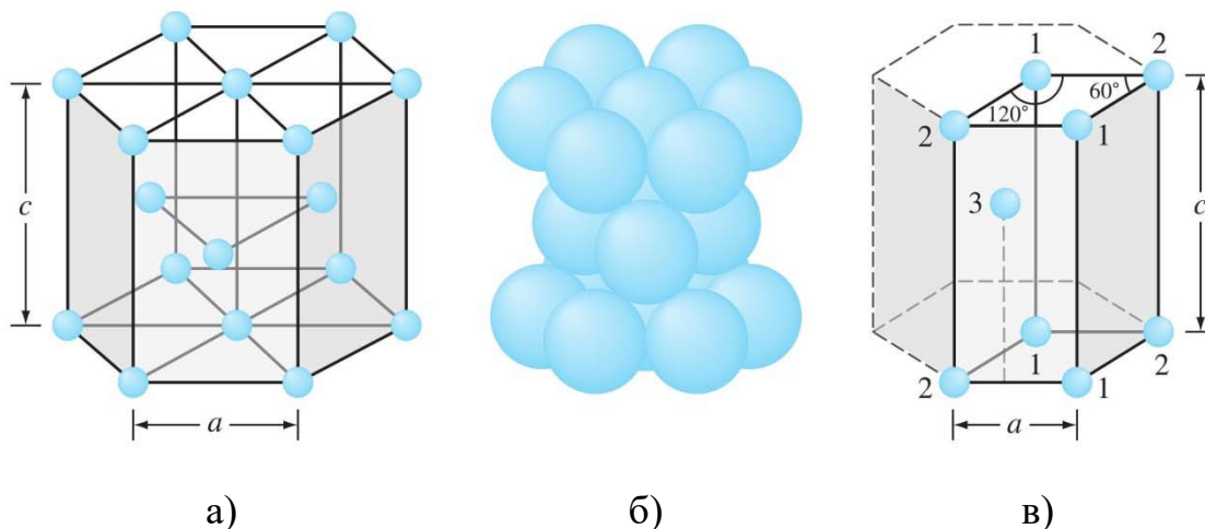
Рис. 3.9. Кристалічна структура ГЦУ ґратки: а) – схема кристалічної структури; б) – модель твердої сфери; в) – схема ізольованої елементарної комірки.
