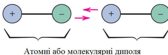
Рис. 2.12. Схематична ілюстрація Ван-дер-Ваальсового зв'язку між двома диполями.
