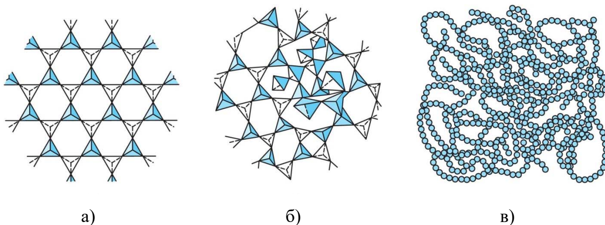
Рис. 3.30. Схема, що показує різні ступені впорядкованості матеріалів: а) – дальній порядок у кристалічному кремнеземі; б) – кварцове скло без дальнього порядку; в) – аморфна структура в полімерах.
