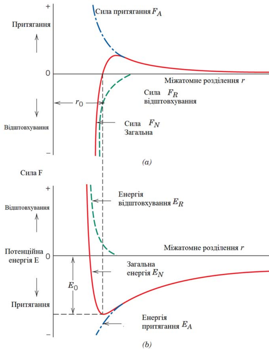
Рис. 2.8. Залежність сил відштовхування, притягання та взаємодії від міжатомного віддалення для двох ізолюваних атомів( a ) і залежність енергій відштовхування, притягання та чистої потенціальної енергії від міжатомного віддалення для двох ізолюваних атомів ( b ).
