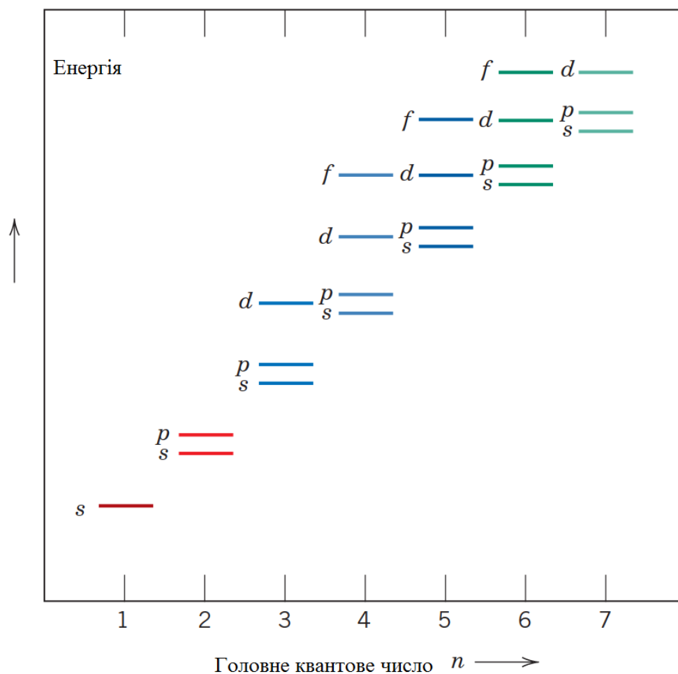
Рис. 2.4. Схематичне зображення відносної енергії електронів для різних оболонок і підоболонки.
