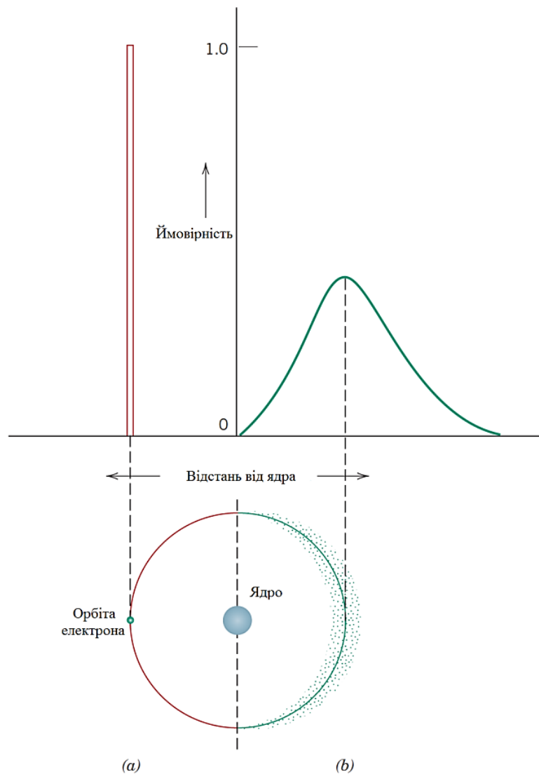
Рис. 2.3. Порівняння борівської (а) та хвильово-механічної (b) моделей атома з точки зору розподілу електронів.
