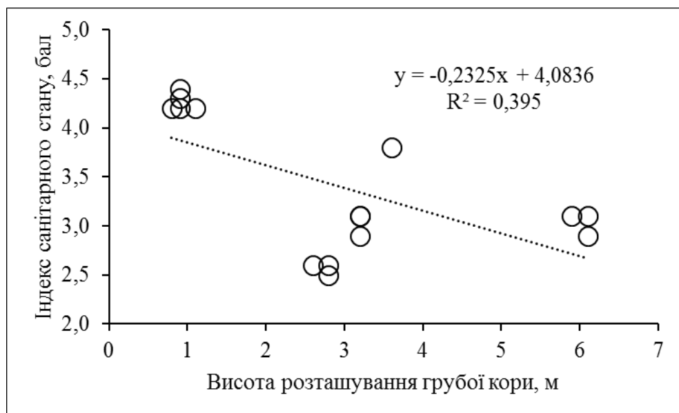
Рис. 3.6. Залежність індексу санітарного стану дерев від висоти розташування верхньої межі грубої кори
