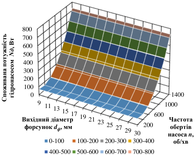
Рис. 2. Залежність потужності N_d , що витрачається на перемішування та циркуляцію емульсії від частоти обертів гідронасоса n та діаметра сопла форсунки d_\phi
