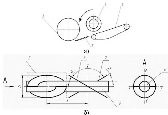
а - схема встановлення розрихлювача-вирівнювача; б - схема робочих органів розрихлювача-вирівнювача; 1 - опорне колесо, 2 - підкопуючий леміш, 3 - прутковий елеватор, 4 - розрихлювач-вирівнювач, 5 - розрихлюючий елемент, 6,7 - півдиски розрихлюючого елемента, 8 - барабан
