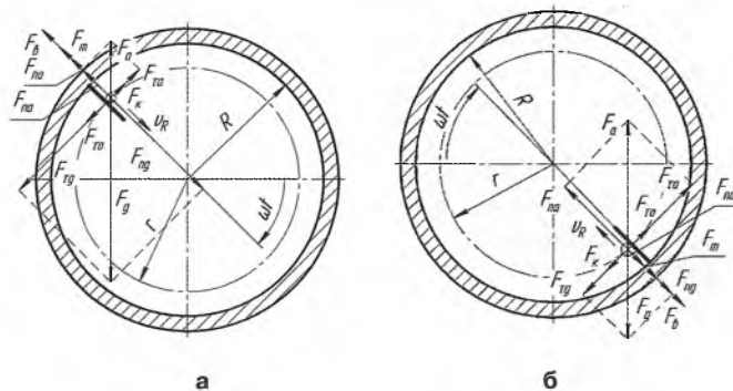
Рис. 1 – Схема дії сил на мінеральні (а) та органічні (б) частинки субстрату F_g – сила тяжіння, Н; F_a – сила Архімеда, Н; F_m – сила тертя, Н; F_k – коріолісова сила інерції, Н; F_b – відцентрова сила інерції, Н; F_{ю} – сила, що притискує частинку до лопатки завдяки опору субстрату, Н; F_{ю0} – сила опору субстрату, яка протидіє руху частинки у радіальному напрямку, Н; r – поточний радіус положення частинки субстрату, м; v_R – відносна швидкість органічної частинки під час руху по лопатці, м/с; R – внутрішній радіус метантенка, м; \omega t – кут повороту метантенка, рад.
