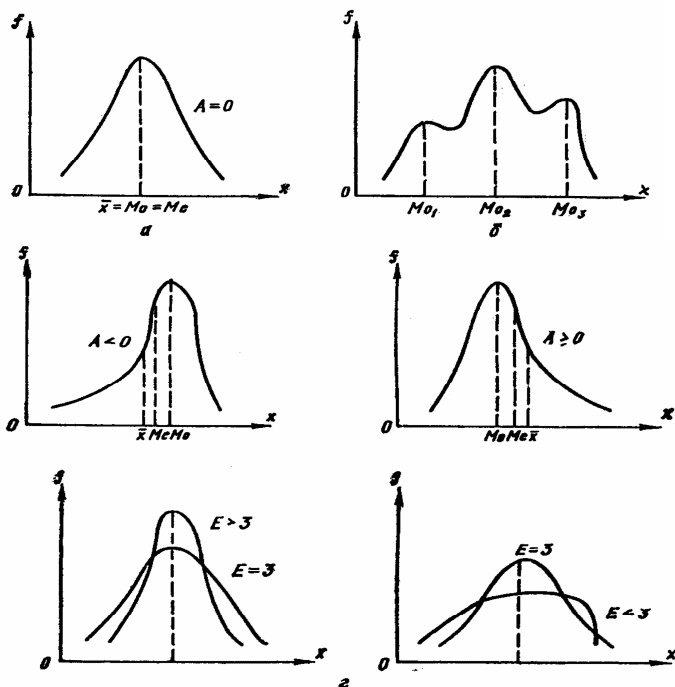
Рис. 2.2.3. Різновиди форм розподілу
