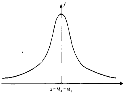
Рис. 2.2.4. Крива нормального розподілу
