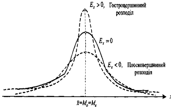
Рис. 2.2.2. Ексцес розподілу
