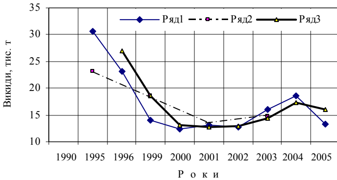
Рис. 2.6.2. Згладжування рядів динаміки
