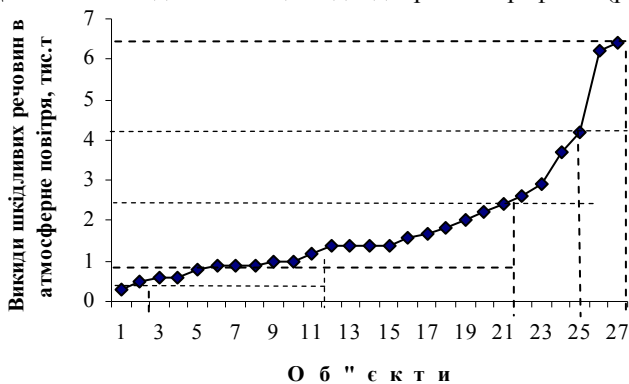
Рис. 2.2. Огіва ранжируваного ряду
