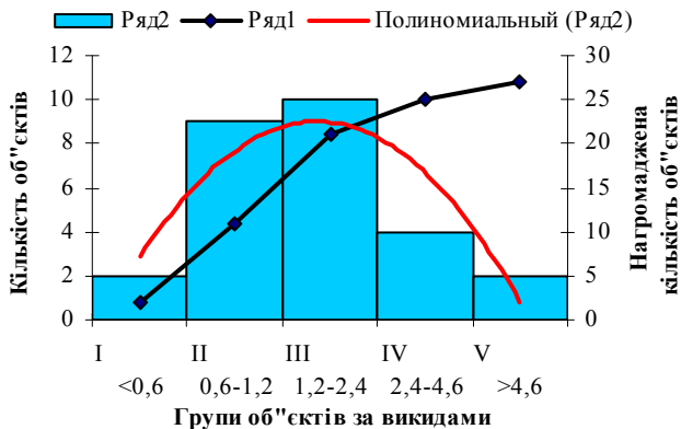
Рис. 2.1.5. Гістограма розподілу об'єктів Житомирщини за викидами, 2005 р.
