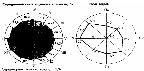
Рис. 1.5.1. Кліматограми
