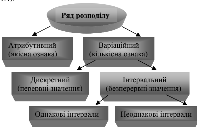
Рис. 2.1.4. Види рядів розподілу
