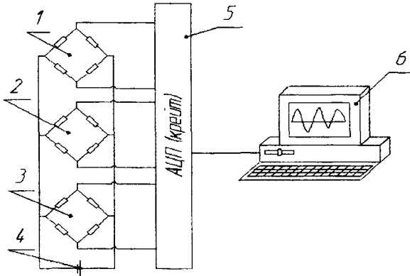
Рис. 4. Блок-схема вимірювально-реєструючої апаратури установки для дослідження зчипних властивостей моделі еластичної шини з ґрунтом: 1 – тензоміст для вимірювання сили зсуву P_s ; 2 – тензоміст для вимірювання навантаження на рейку G_p ; 3 – тензоміст для вимірювання переміщення рейки S_p ; 4 – акумуляторна батарея (12в); 5 – аналого-цифровий перетворювач (АЦП); 6 – комп'ютер
