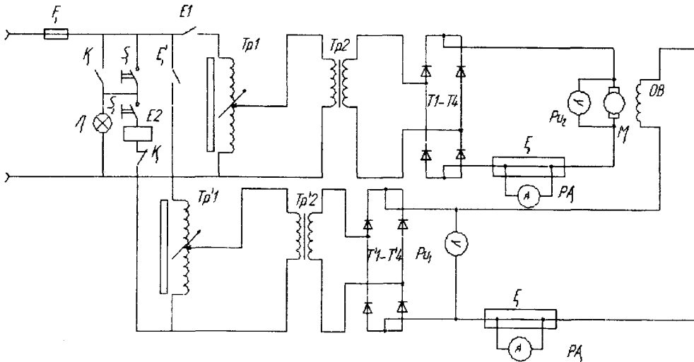
Рис. 5. Електрична схема силового приводу стенда
