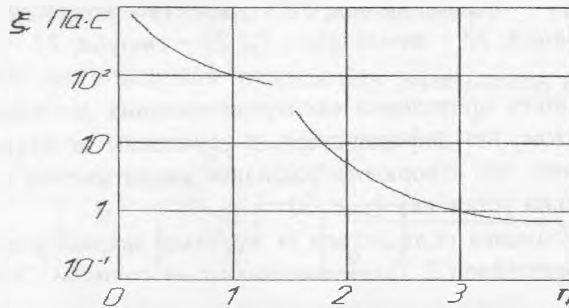
Рис. 2. Залежність вібров'язкості піску від прискорення вібрації
