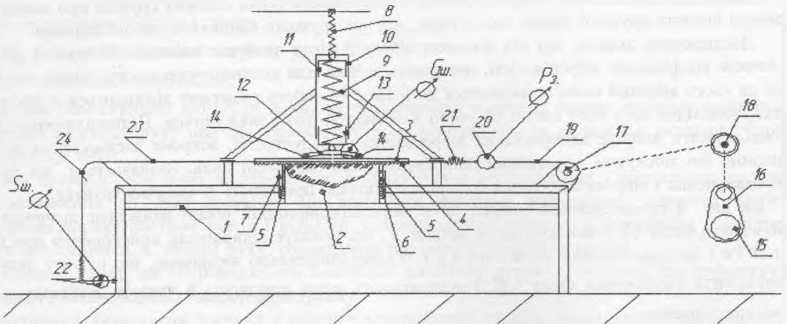
Рис. 3. Експериментальна установка для дослідження зчіпних властивостей моделі шини з ґрунтом: 1 – рама; 2 – контейнер з ґрунтом; 3 – рейка; 4 – модель протектора; 5 – шторки; 6 – ролик шторки; 7 – напрямна шторки; 8 – гвинтовий пристрій; 9 – пружина вертикального навантажування; 10 – циліндр; 11 – верхній стакан; 12 – каретка; 13 – нижній стакан; 14 – ролик каретки; 15 – електродвигун; 16 – редуктор; 17 – приводний вал; 18 – шків; 19 – трос; 20 – тензо-ланка P_2 ; 21 – пружна ланка; 22 – тензоланка S_p ; 23 – струна; 24 – напрямна ланка
