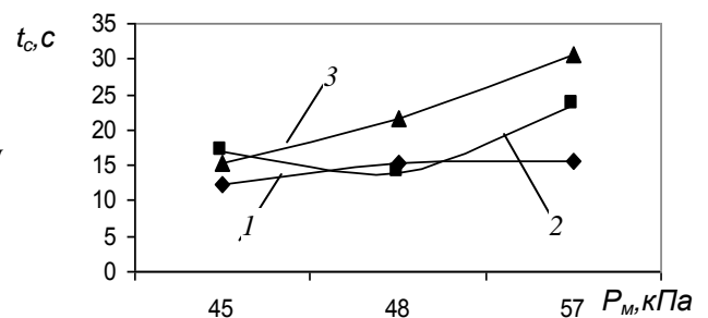
Рис.2. Тривалість стабілізаційного періоду ( t_c ) залежно від рівня магістрального вакуумметричного тиску ( P_m ) при об'ємі вакуумного балона: 1 - без балона; 2 - 0,01 м³; 3 - 0,02 м³
