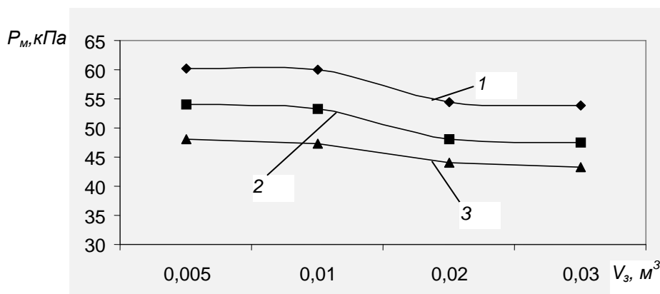
Рис.3. Вплив об'єму ( V_3 ) на зміну вакуумметричного тиску ( P_m ) у доїльному агрегаті при початкових рівнях розрідження ( P_n ): 1 – 60 кПа; 2 – 54 кПа; 3 – 48 кПа
