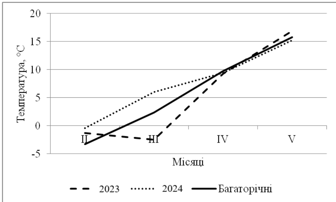
Рис. 3.8 Хід температури повітря весною у 2023, 2024 рр. і за багаторічними даними (м/с Житомир)
