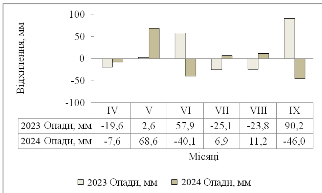
Рис. 3.10 Відхилення кількості опадів у роки досліджень від багаторічних даних
