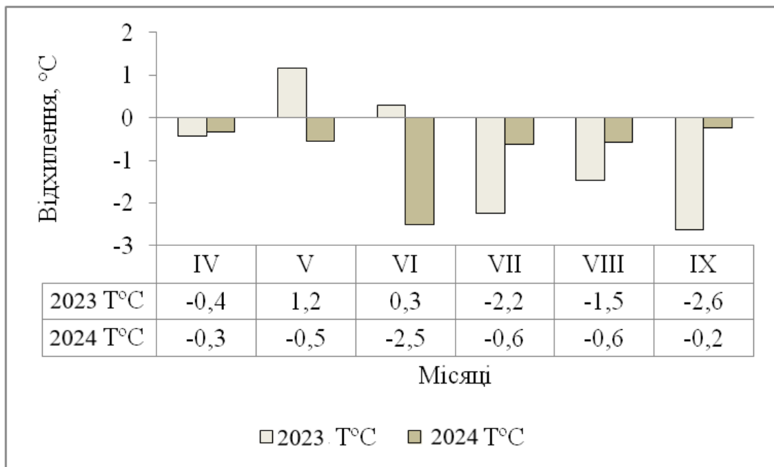
Рис. 3.9 Відхилення температури у роки досліджень від багаторічних даних
